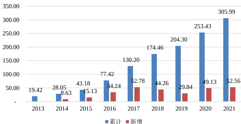
2013-2021年中国光伏发电累计装机量（GW）
