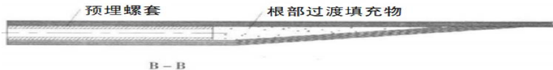
图 4：“预埋螺套”预埋剖面示意图
