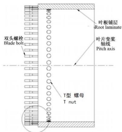
图 1：“T 型螺母”连接方式示意图
