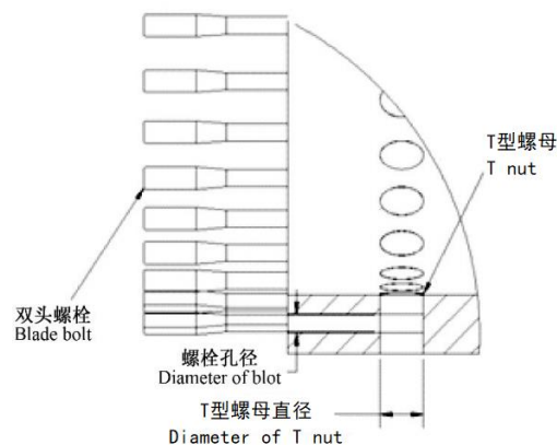
图 2：“T 型螺母”连接细节图
