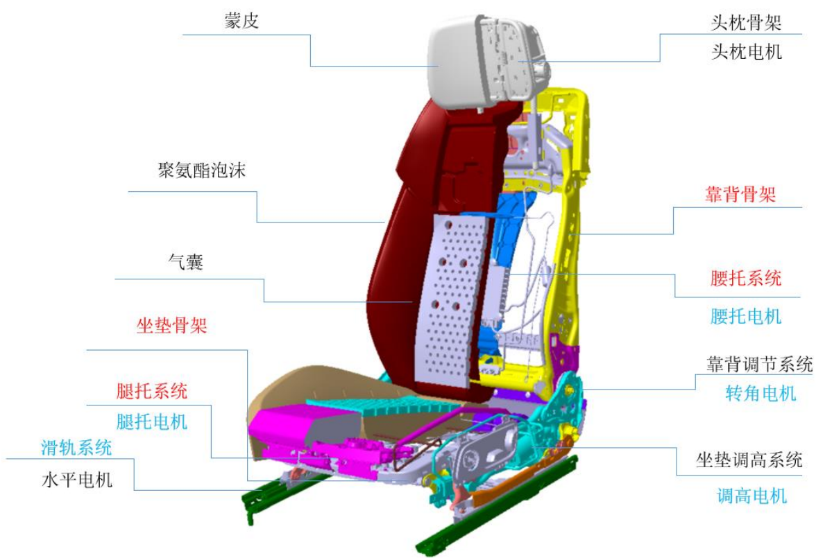
汽车座椅结构图
