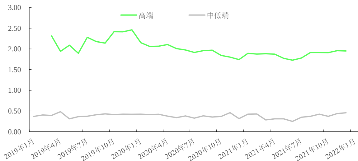
2019-2021 年公司采购英飞凌 MEMS 芯片月度价格变动情况（单位：元/颗）
