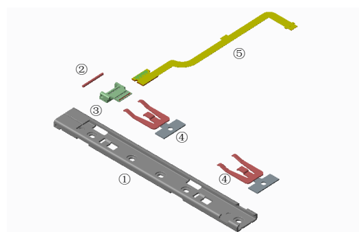
母端滑轨结构:
