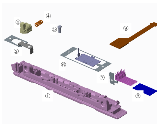
公端滑轨结构:
