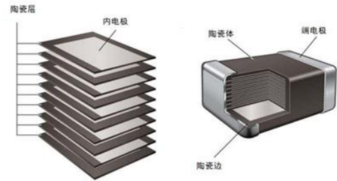
MLCC 内部结构
