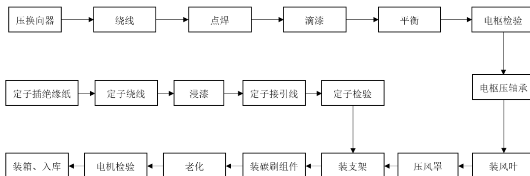
发热芯生产流程图
