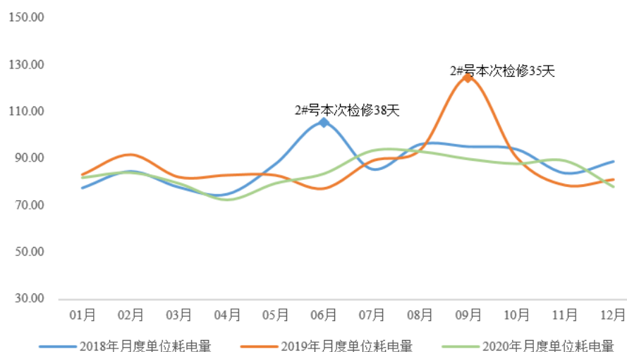
报告期内月度单位耗电量变化（千瓦时/吨）
