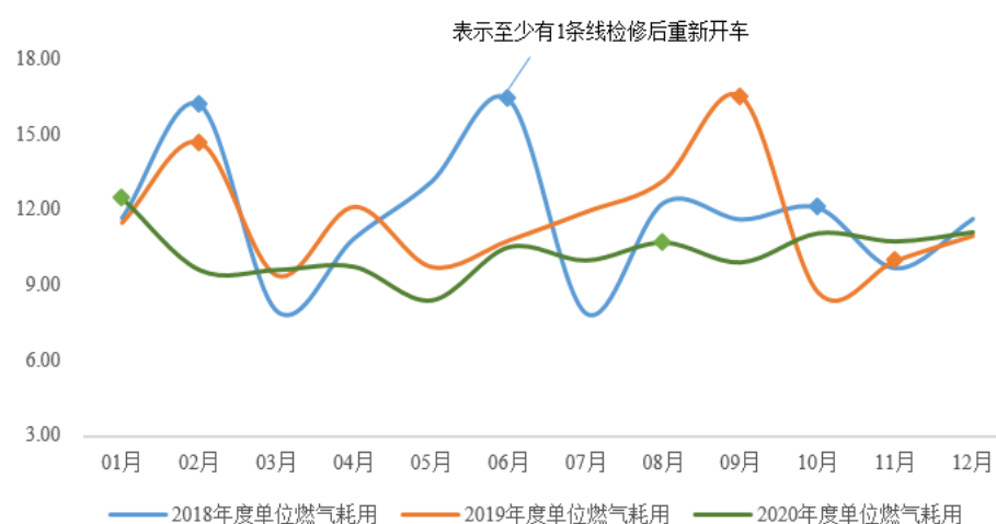
报告期内单位天然气耗用变化（立方米/吨）
