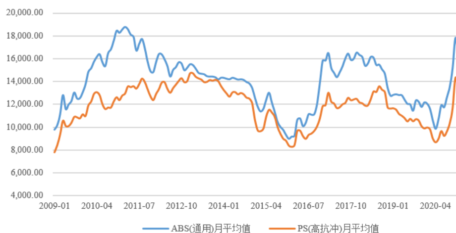
2012年~2020年ABS和HIPS月度均价对比(元/吨)
