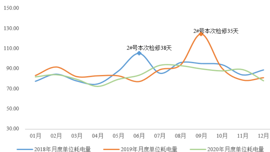
报告期内月度单位耗电量变化（千瓦时/吨）
