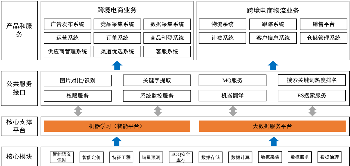
图：公司“大中台”战略架构
