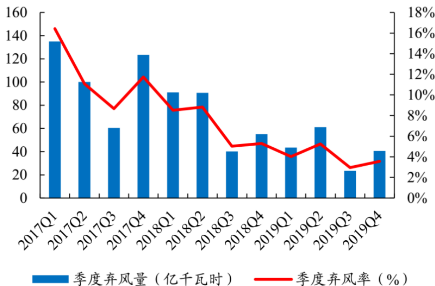
图：我国弃风量及弃风率季度变化
