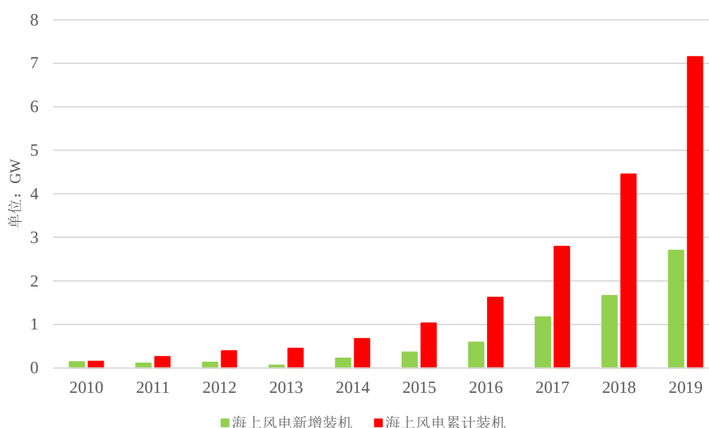
2010-2019年我国海上风电装机容量
