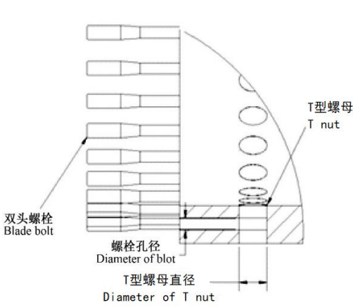
图 2：“T 型螺母”连接细节图
