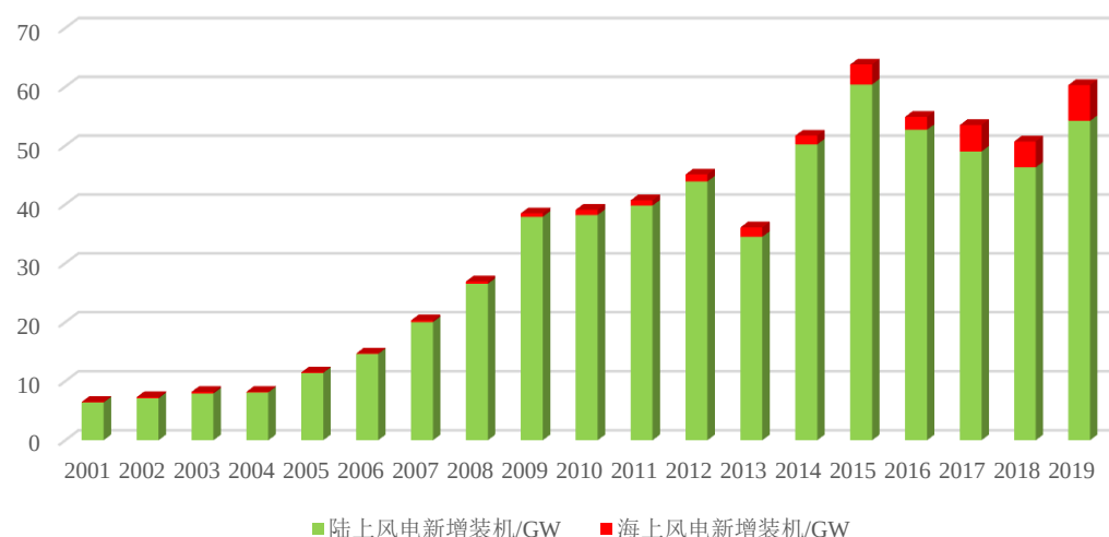
2001年-2019年全球风电新增装机
