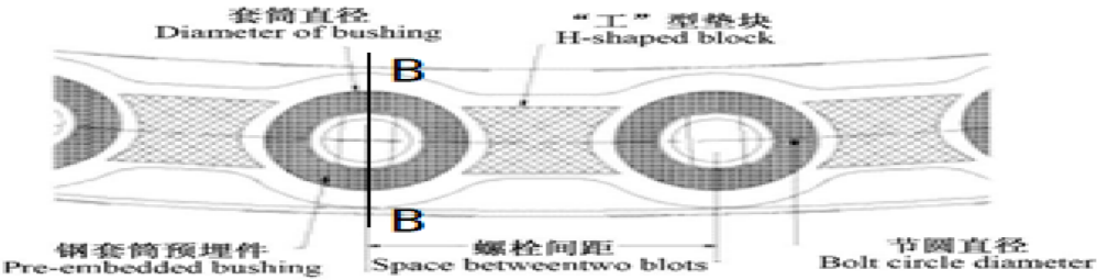
图 3：“预埋螺套”连接细节图
