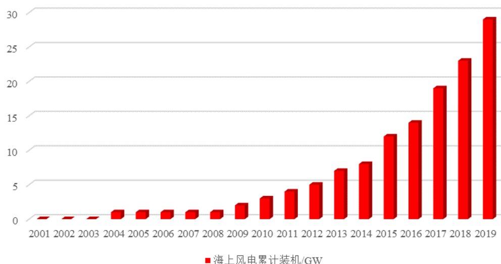
2001年-2019年全球海上风电累计装机
