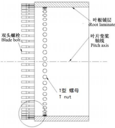
图 1：“T 型螺母”连接方式示意图
