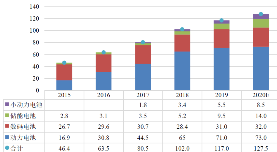
2015-2020 年中国各终端锂电池出货量及预测（单位:GWh）
