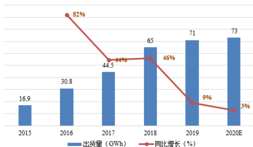
2015-2020 年中国动力电池出货量（单位:GWh）
