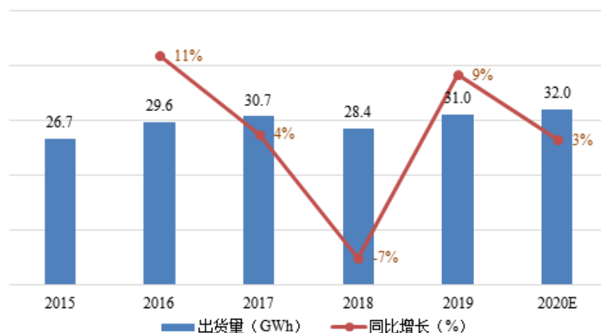
2015-2020 年中国数码电池出货量及预测（单位:GWh）
