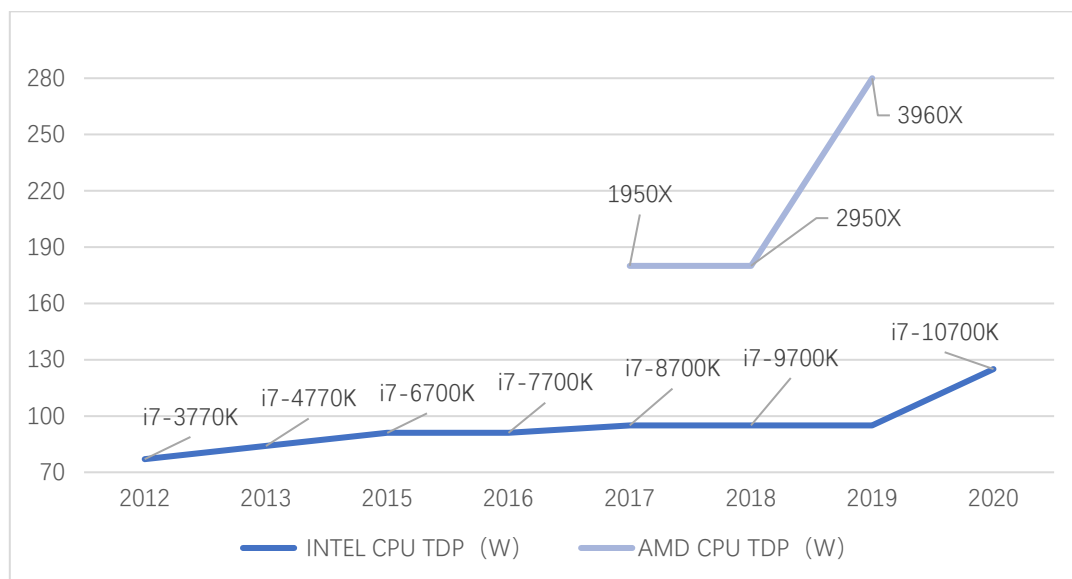
近年来主流 CPU 散热设计功耗变化图
